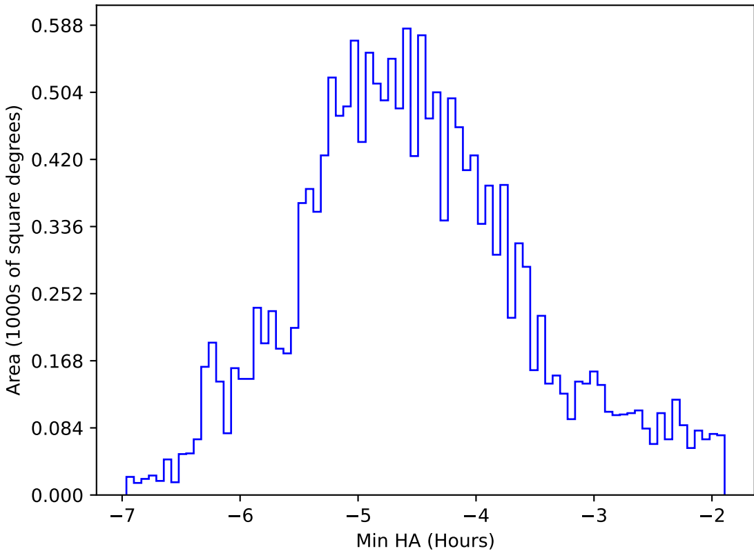
weather_cloudso10v3.4_10yrs WFD i band: Min HA
