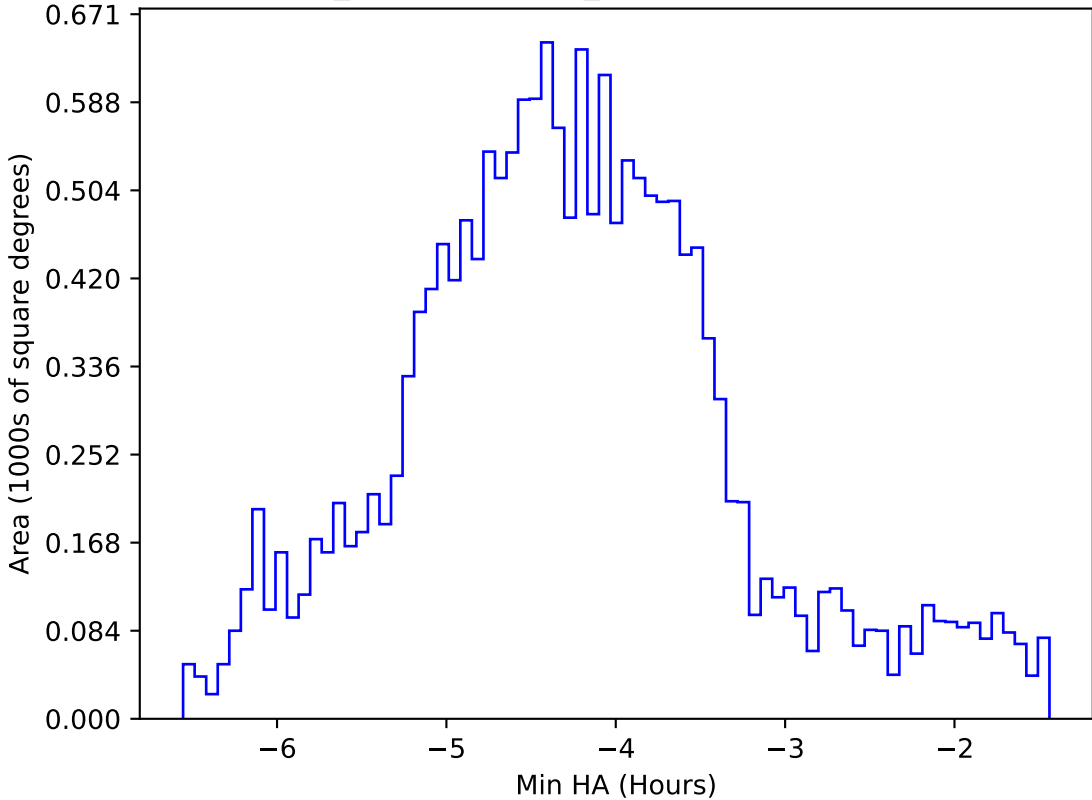
weather_cloudso10v3.4_10yrs WFD g band: Min HA
