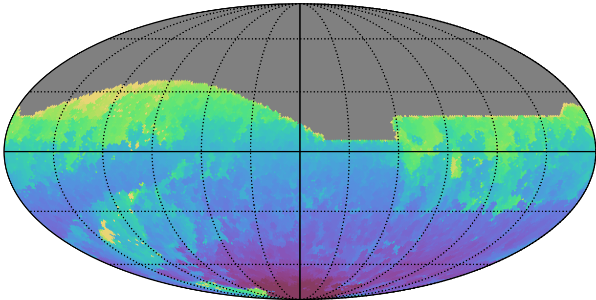
weather_cloudso10v3.4_10yrs All sky z band: Min HA
