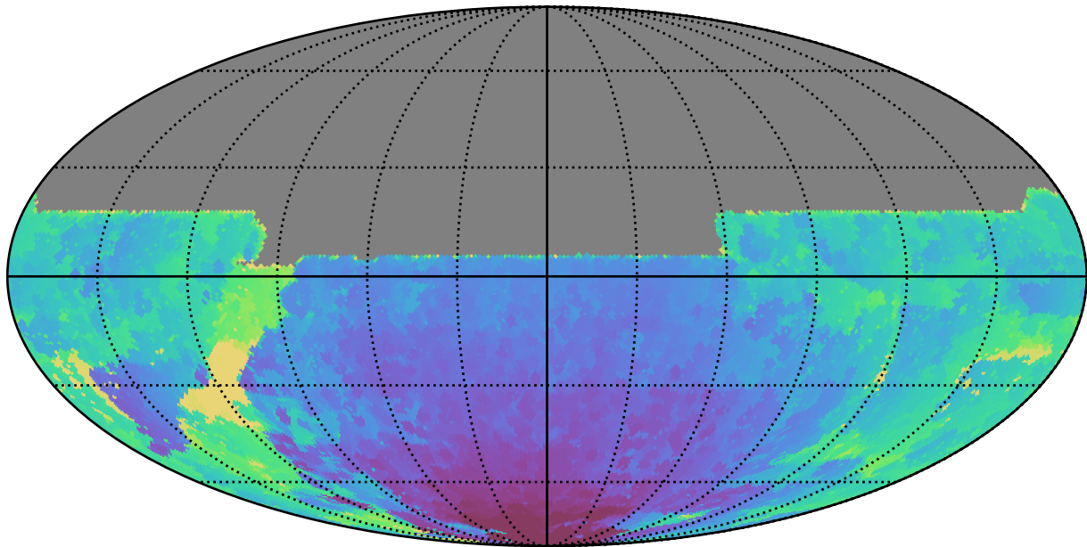
weather_cloudso10v3.4_10yrs All sky y band: Min HA
