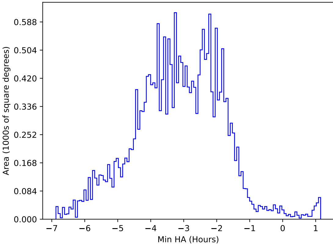
weather_cloudso10v3.4_10yrs All sky u band: Min HA
