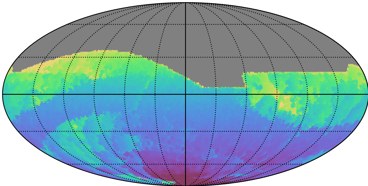
weather_cloudso10v3.4_10yrs All sky r band: Min HA
