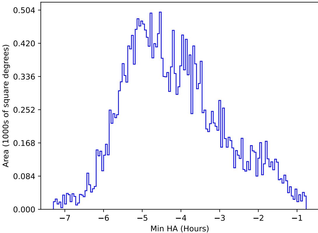
weather_cloudso10v3.4_10yrs All sky r band: Min HA
