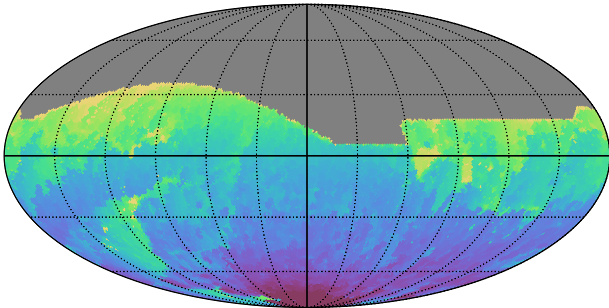
weather_cloudso10v3.4_10yrs All sky i band: Min HA
