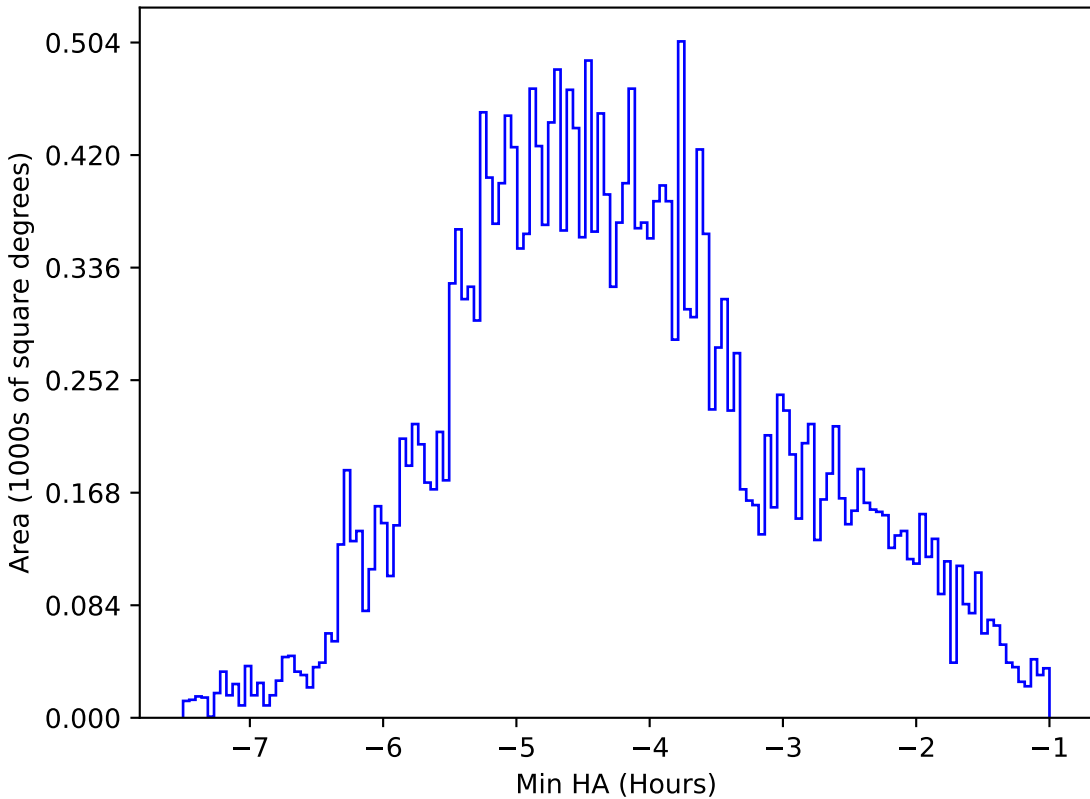
weather_cloudso10v3.4_10yrs All sky i band: Min HA
