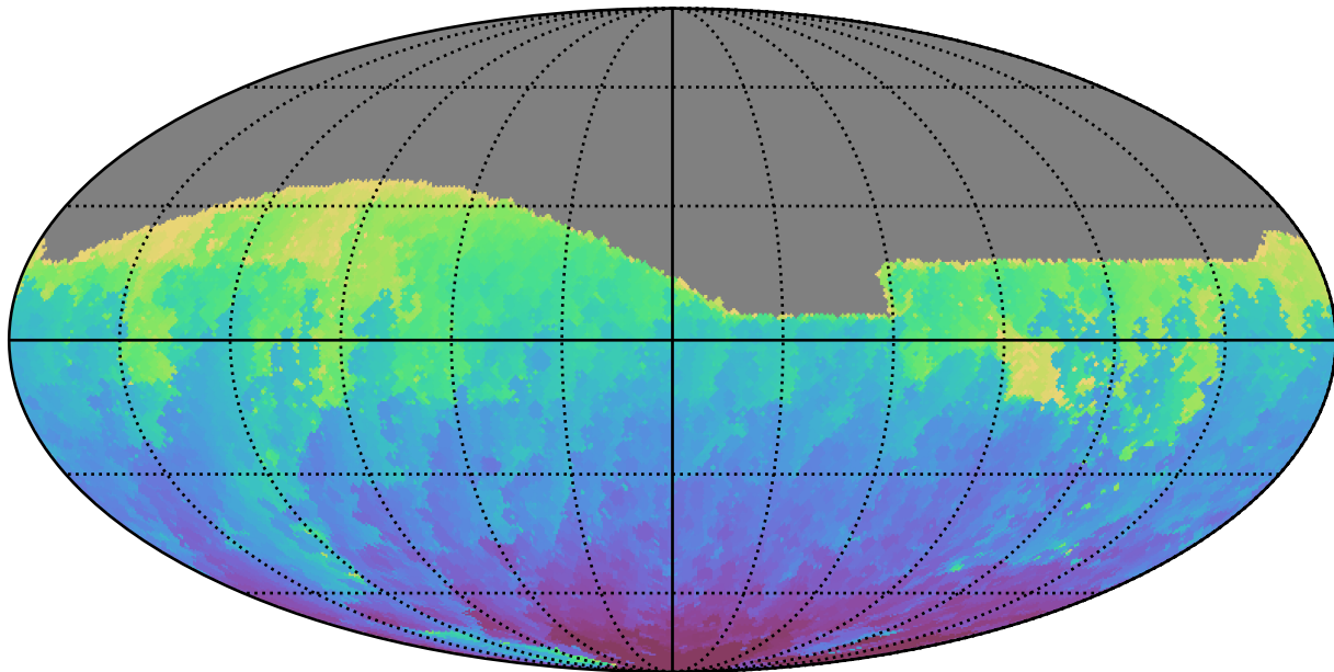
weather_cloudso10v3.4_10yrs All sky g band: Min HA
