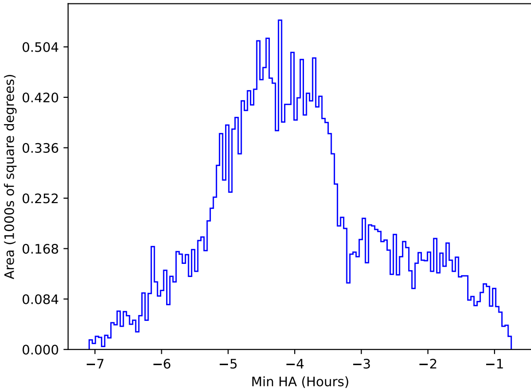
weather_cloudso10v3.4_10yrs All sky g band: Min HA
