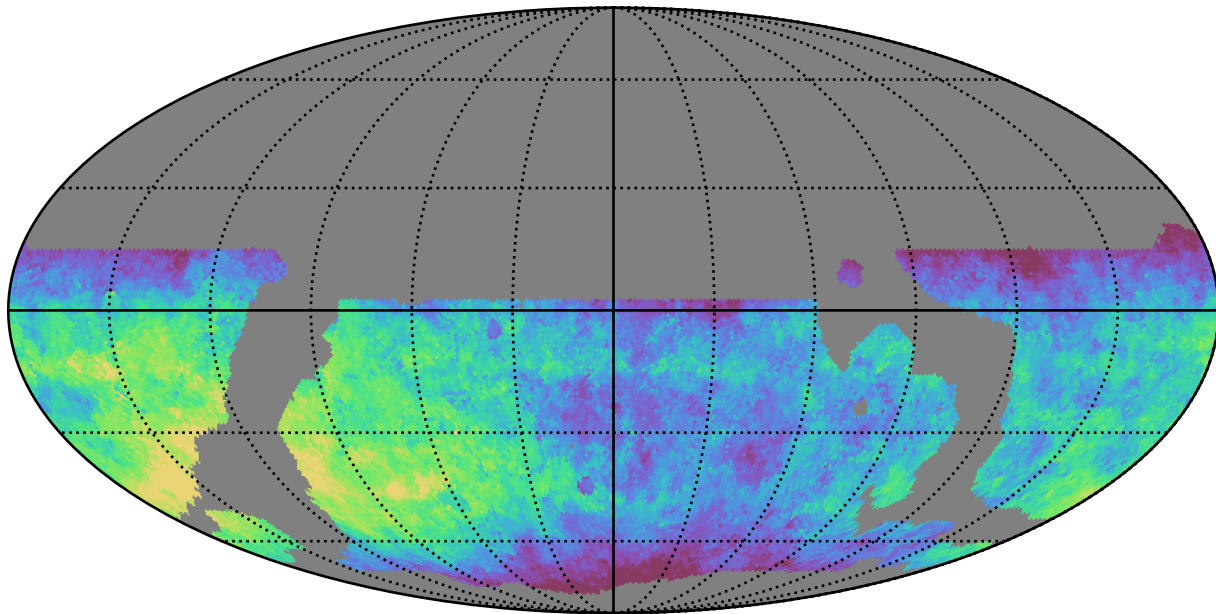
weather_cloudso10v3.4_10yrs WFD z band: Median saturation_mag
