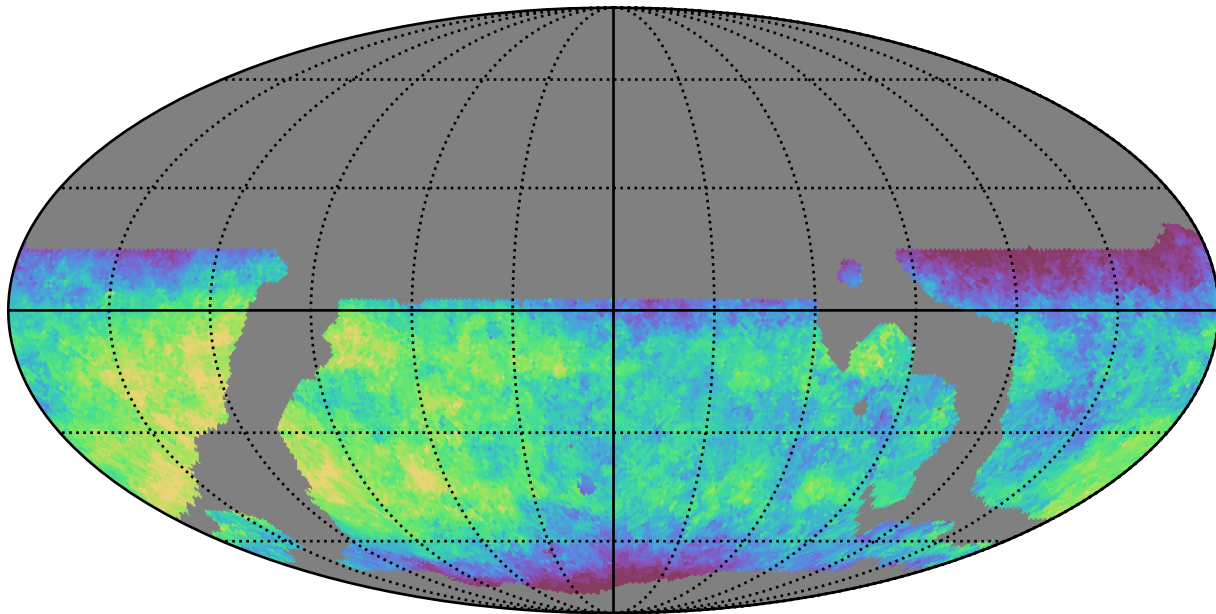
weather_cloudso10v3.4_10yrs WFD y band: Median saturation_mag
