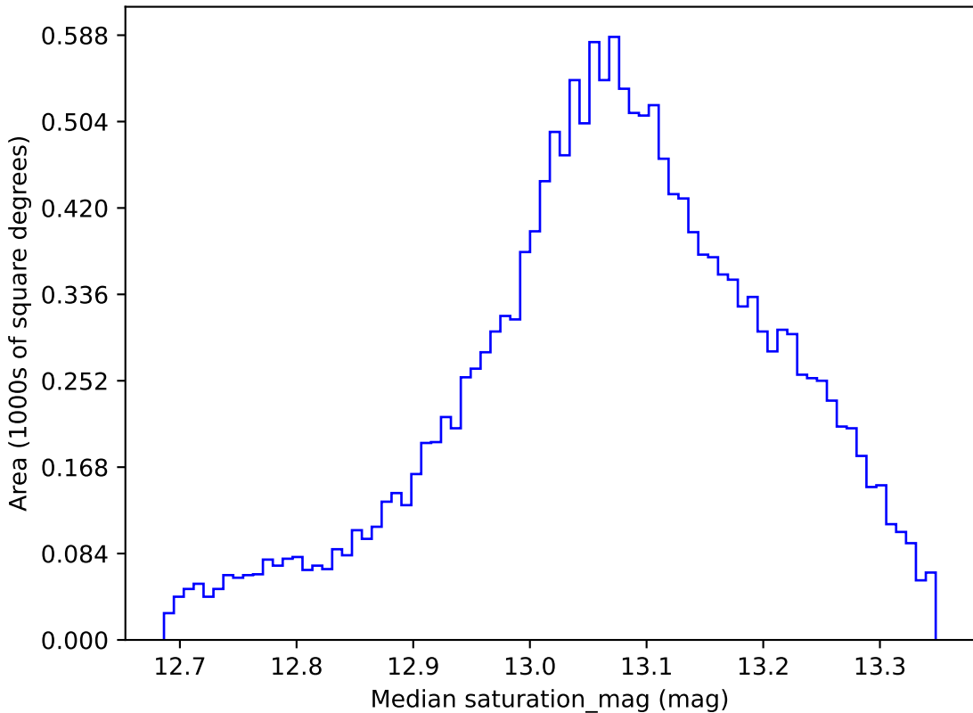
weather_cloudso10v3.4_10yrs WFD y band: Median saturation_mag
