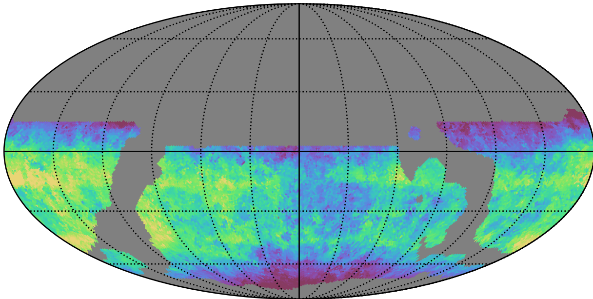
weather_cloudso10v3.4_10yrs WFD g band: Median saturation_mag
