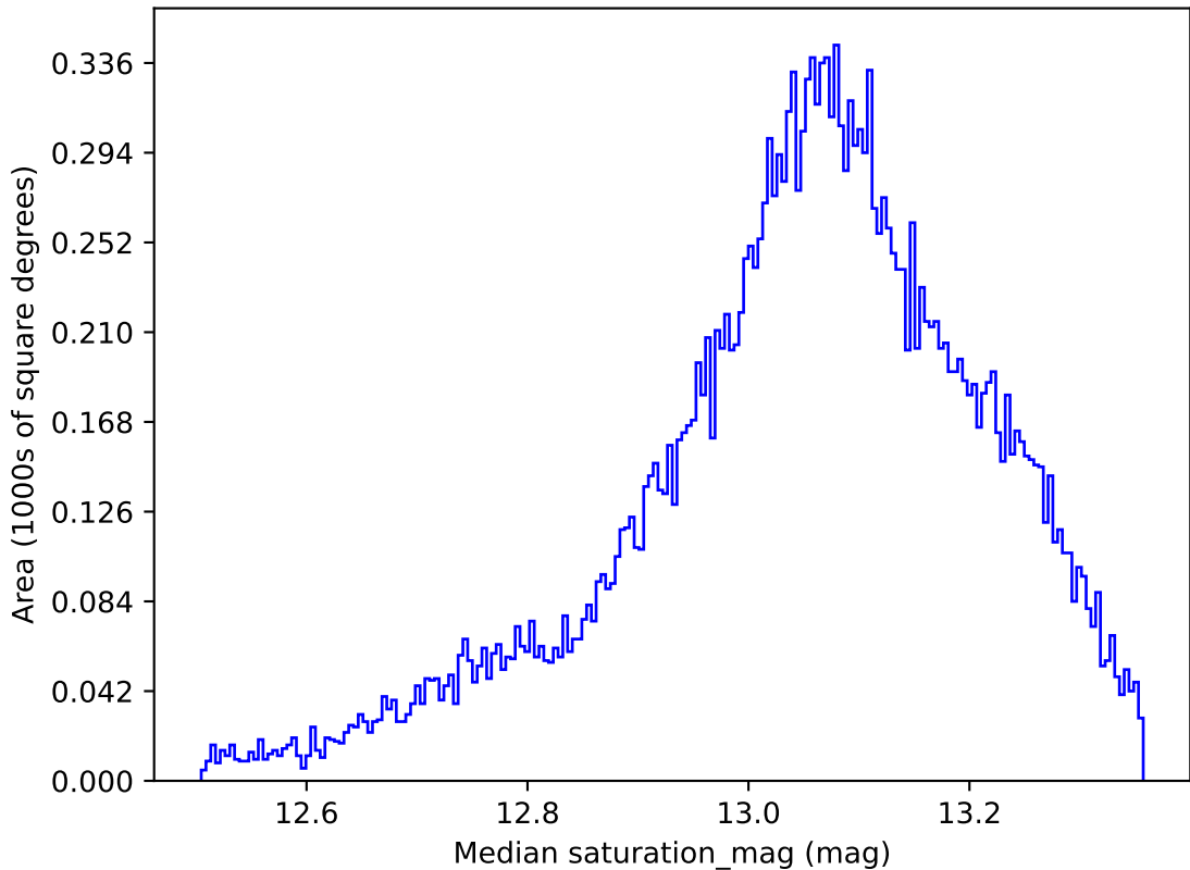
weather_cloudso10v3.4_10yrs All sky y band: Median saturation_mag
