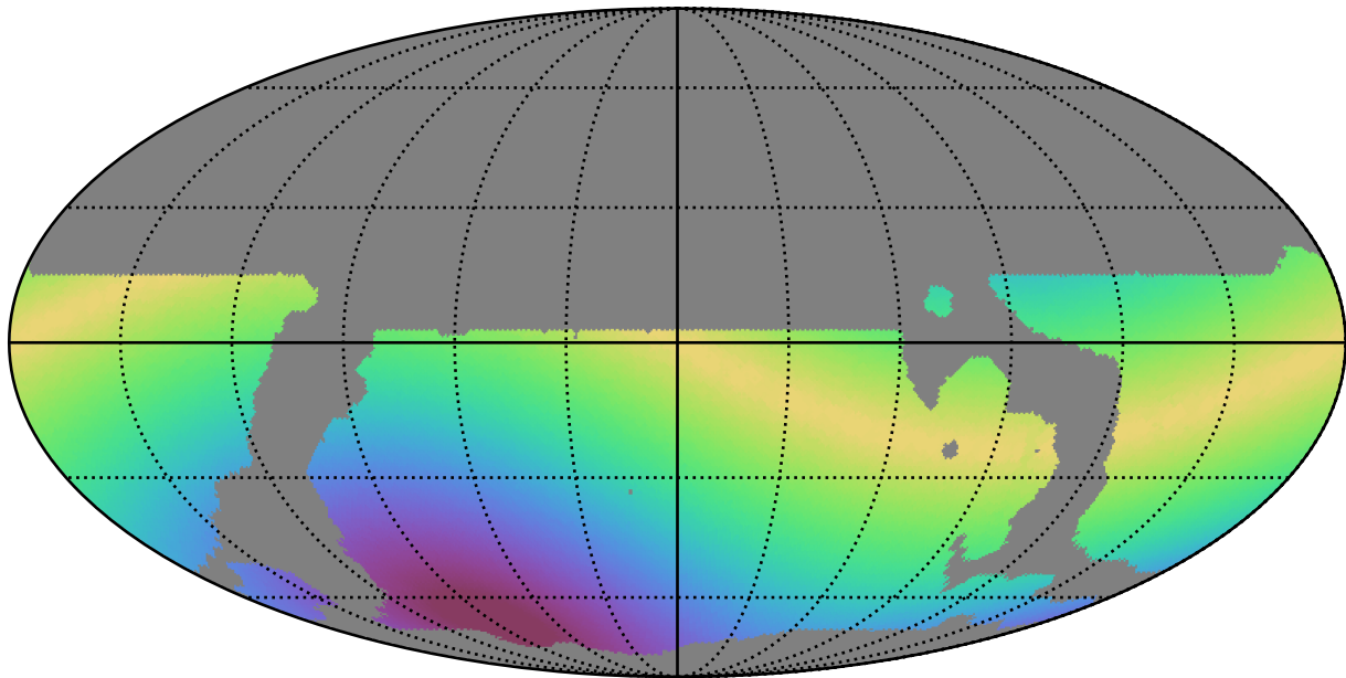
weather_cloudso10v3.4_10yrs WFD i band: Max solarElong
