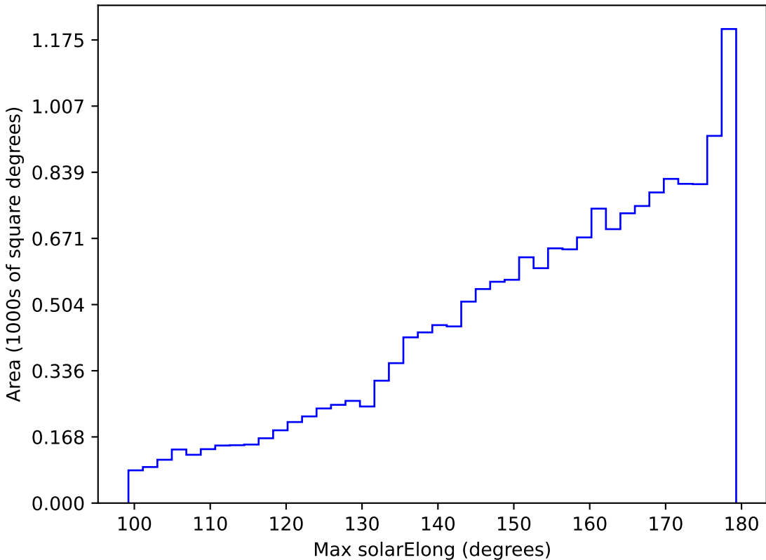
weather_cloudso10v3.4_10yrs WFD i band: Max solarElong
