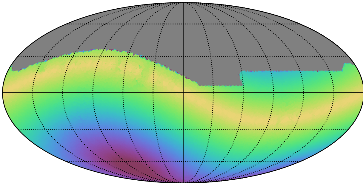
weather_cloudso10v3.4_10yrs All sky i band: Max solarElong
