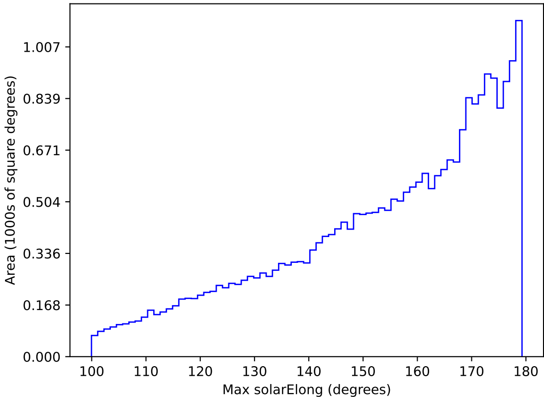
weather_cloudso10v3.4_10yrs All sky i band: Max solarElong
