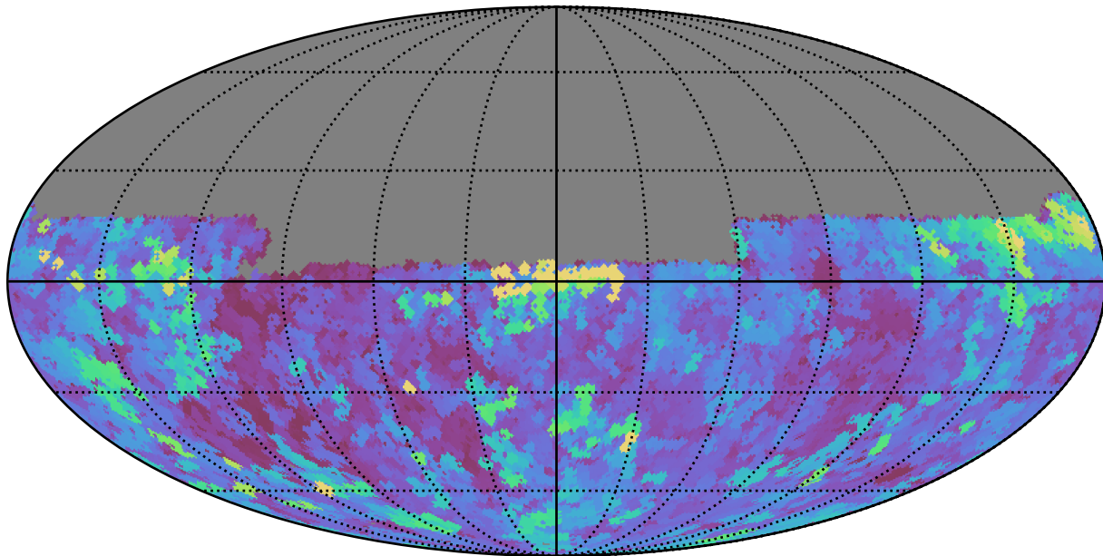
weather_cloudso10v3.4_10yrs Yr 1 y band: Max seeingGeom
