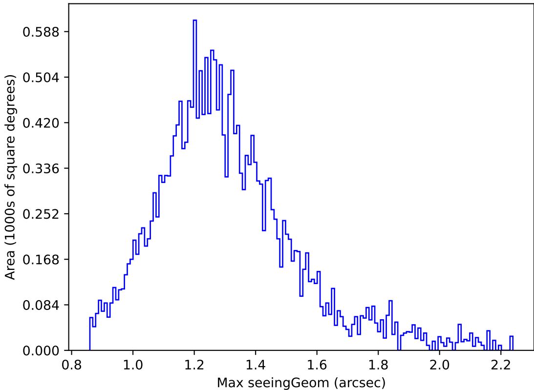
weather_cloudso10v3.4_10yrs Yr 1 y band: Max seeingGeom
