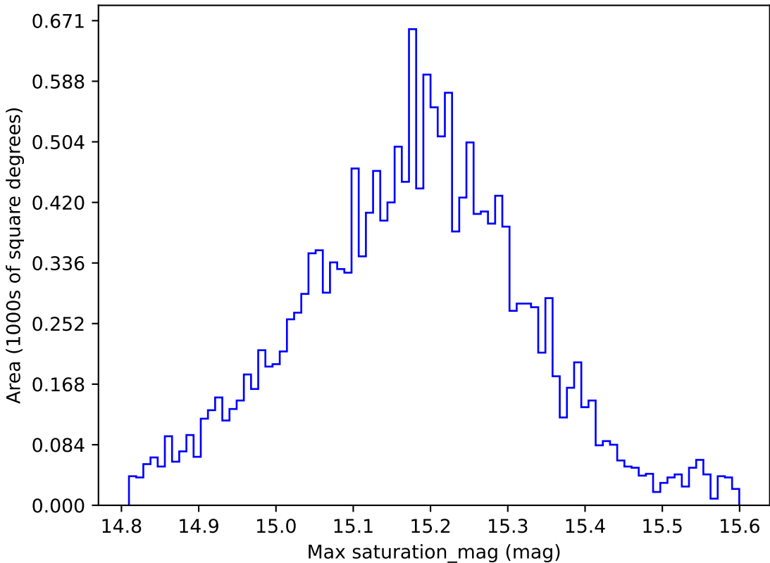
weather_cloudso10v3.4_10yrs WFD z band: Max saturation_mag
