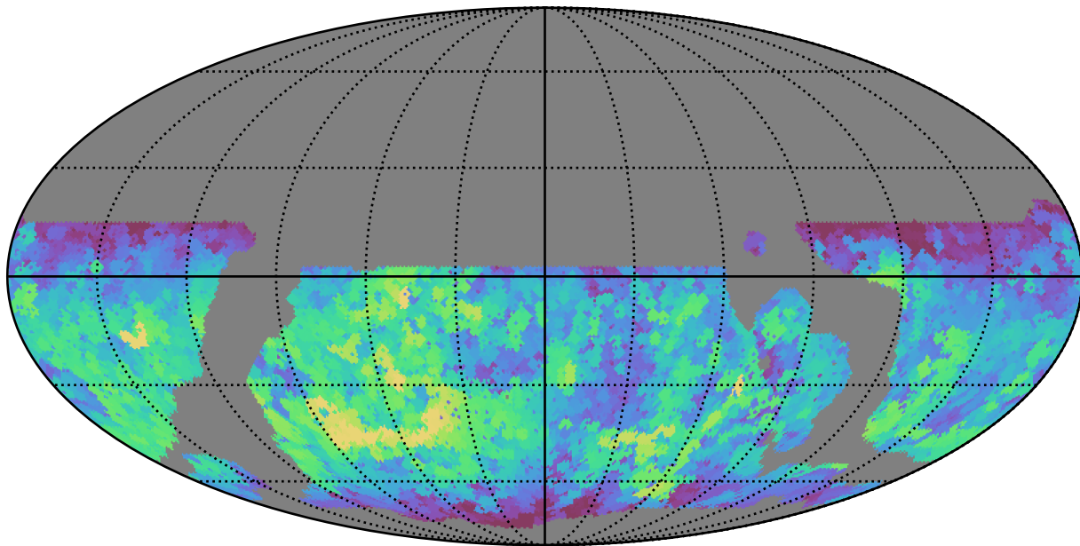
weather_cloudso10v3.4_10yrs WFD y band: Max saturation_mag
