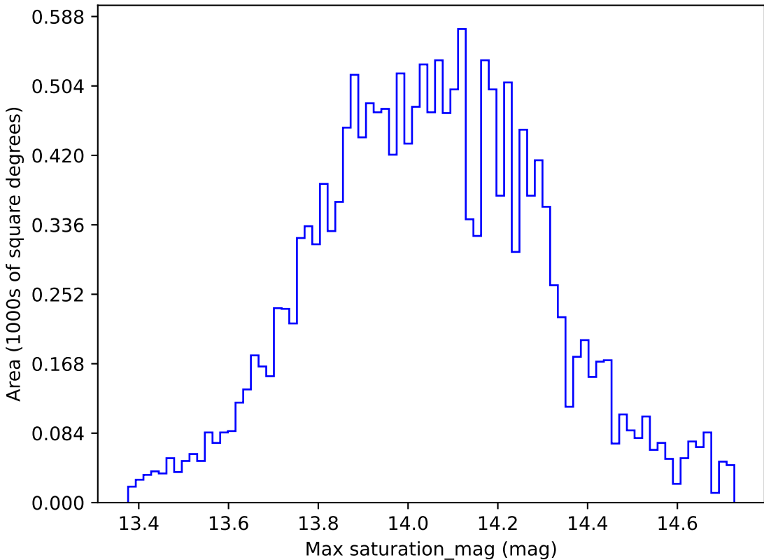
weather_cloudso10v3.4_10yrs WFD u band: Max saturation_mag
