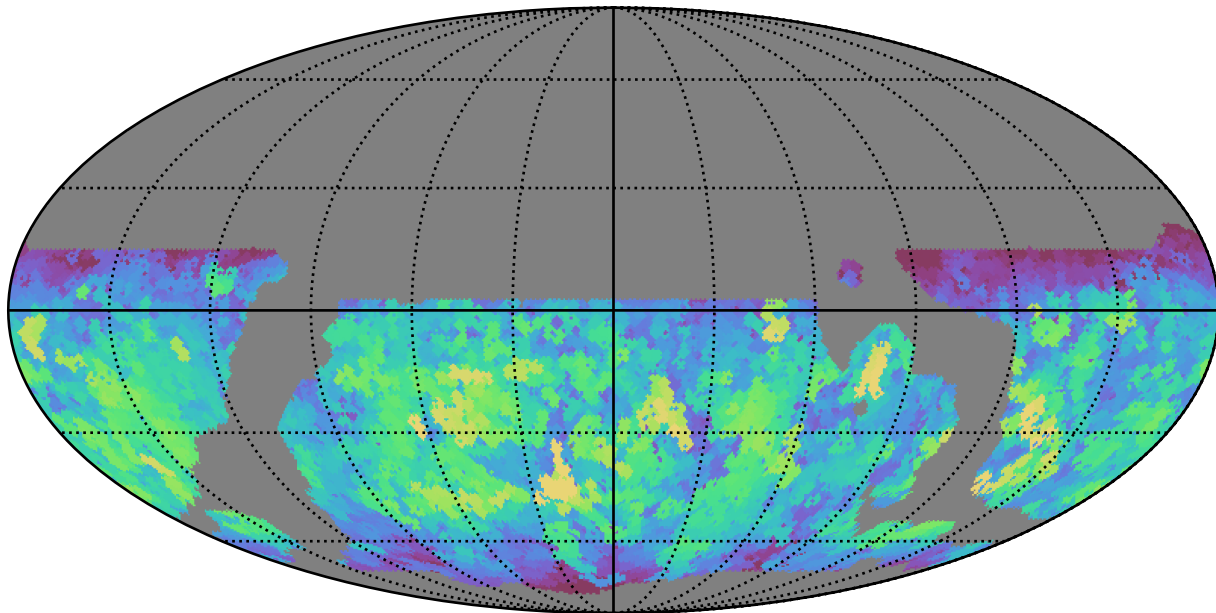
weather_cloudso10v3.4_10yrs WFD r band: Max saturation_mag
