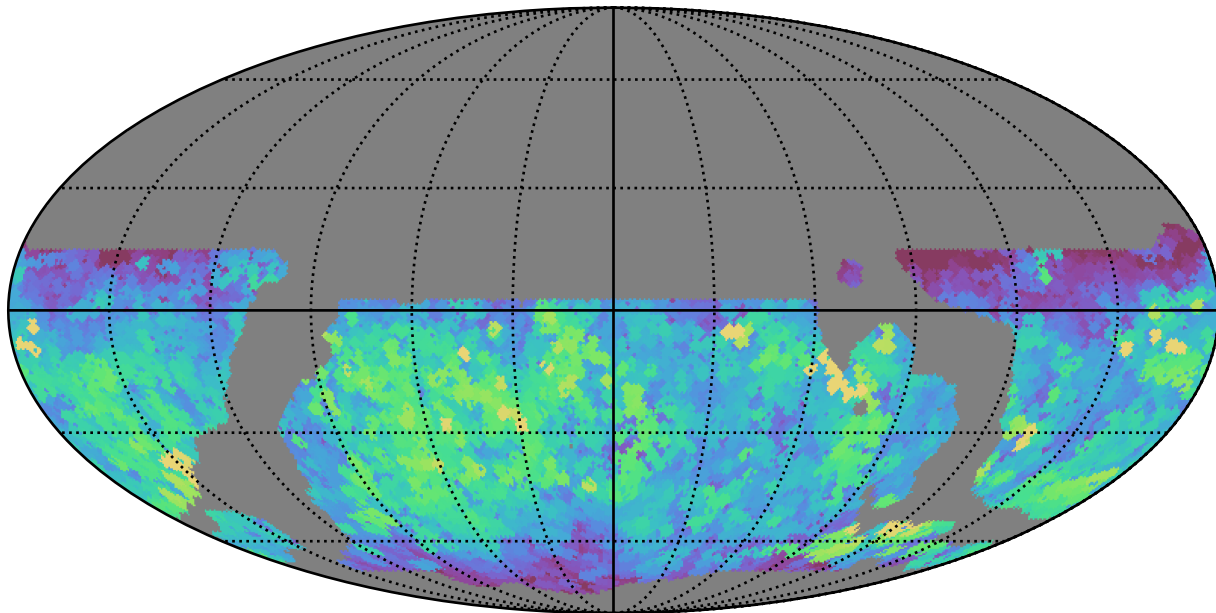
weather_cloudso10v3.4_10yrs WFD i band: Max saturation_mag
