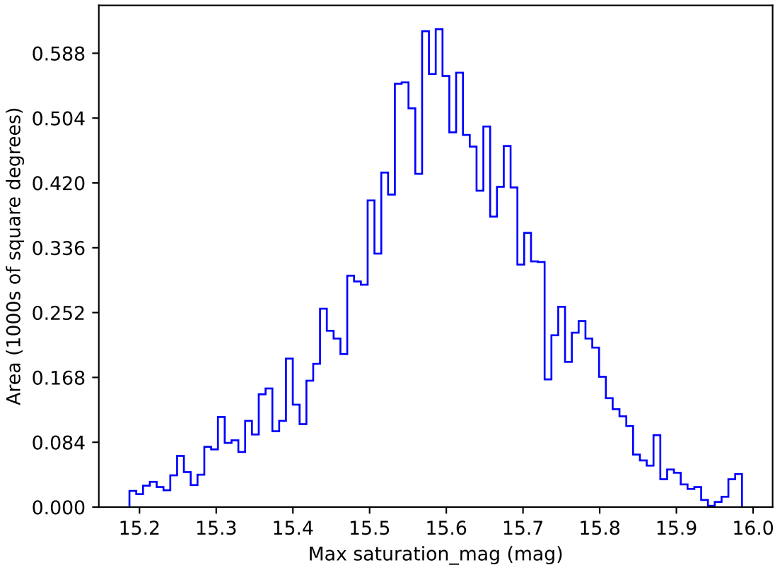
weather_cloudso10v3.4_10yrs WFD i band: Max saturation_mag
