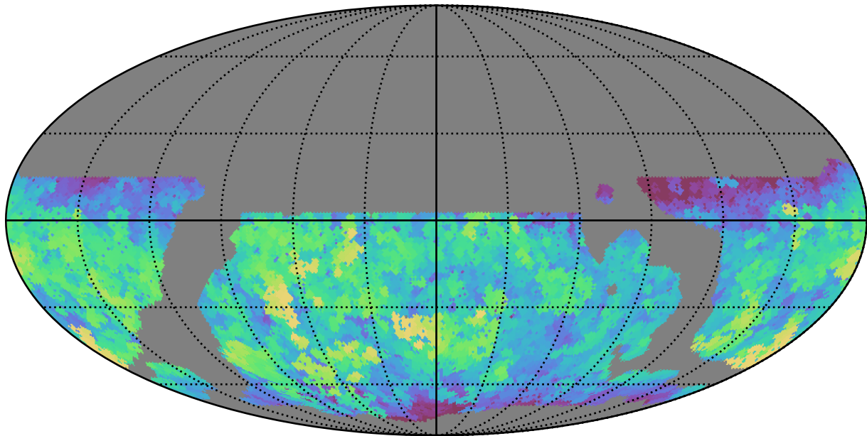
weather_cloudso10v3.4_10yrs WFD g band: Max saturation_mag
