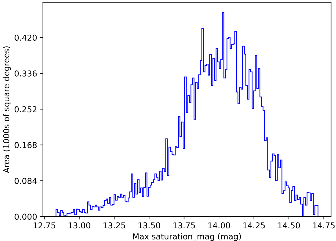
weather_cloudso10v3.4_10yrs All sky u band: Max saturation_mag
