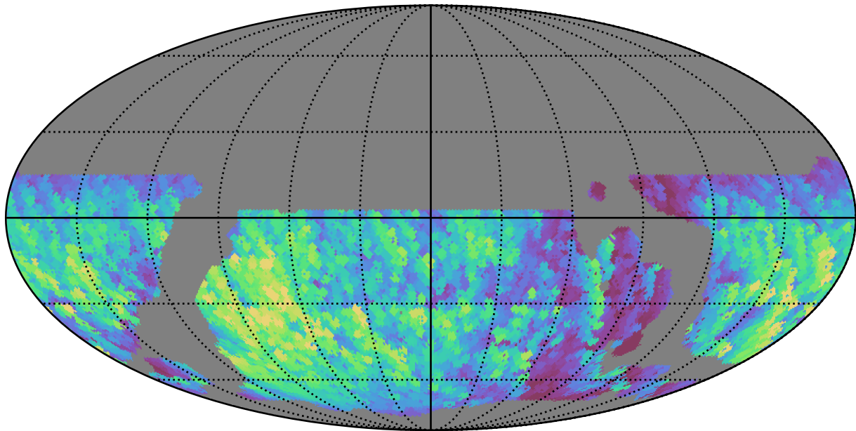
weather_cloudso10v3.4_10yrs WFD y band: Max normairmass
