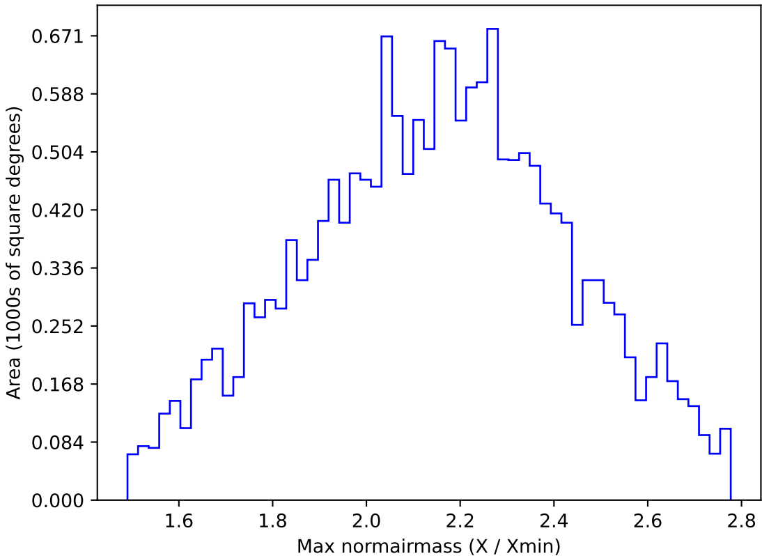
weather_cloudso10v3.4_10yrs WFD y band: Max normairmass
