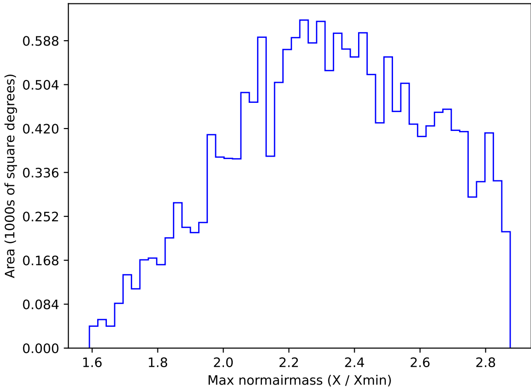
weather_cloudso10v3.4_10yrs WFD i band: Max normairmass
