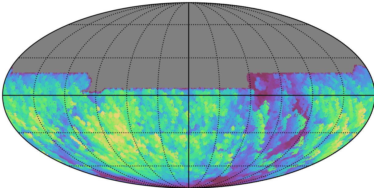
weather_cloudso10v3.4_10yrs All sky y band: Max normairmass
