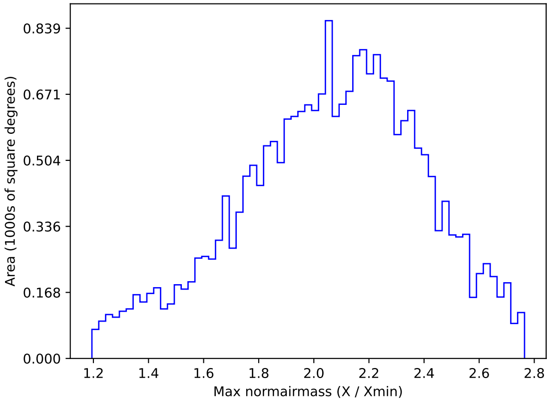
weather_cloudso10v3.4_10yrs All sky y band: Max normairmass
