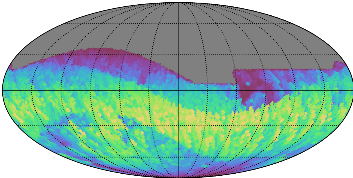
weather_cloudso10v3.4_10yrs All sky i band: Max normairmass
