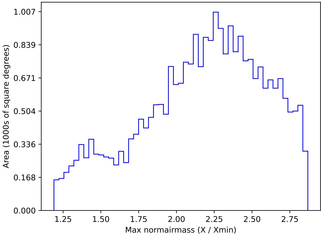
weather_cloudso10v3.4_10yrs All sky i band: Max normairmass
