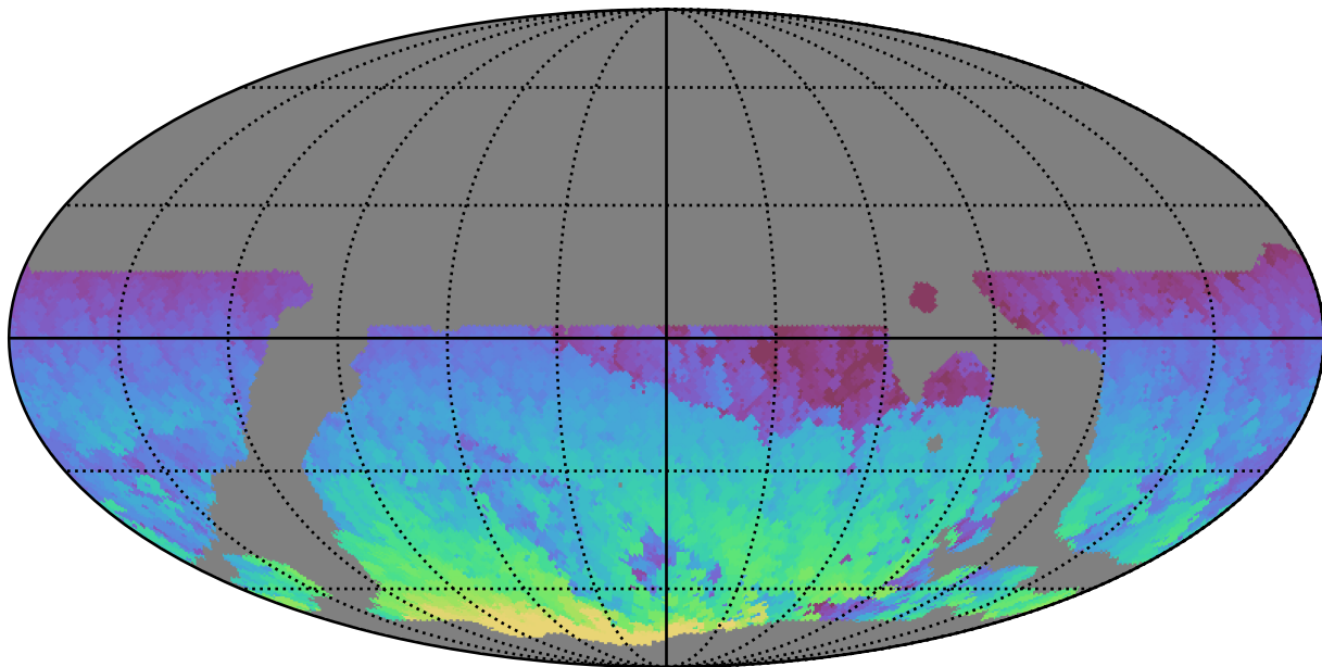
weather_cloudso10v3.4_10yrs WFD z band: Max HA
