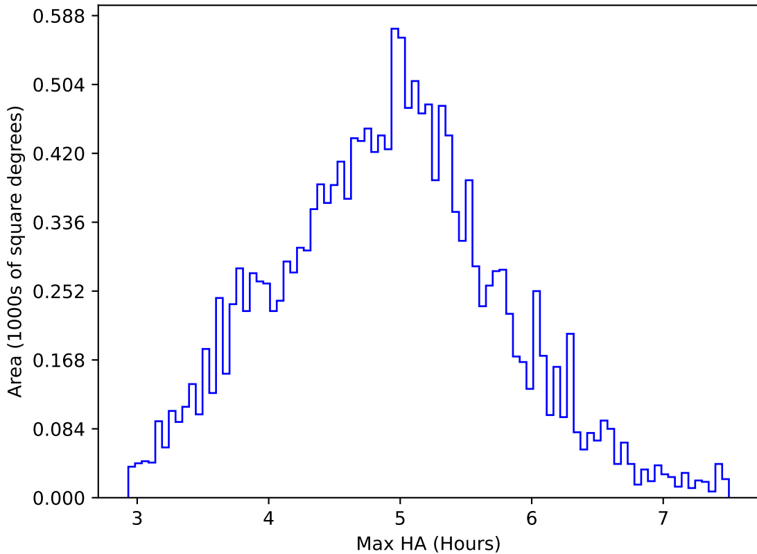
weather_cloudso10v3.4_10yrs WFD z band: Max HA
