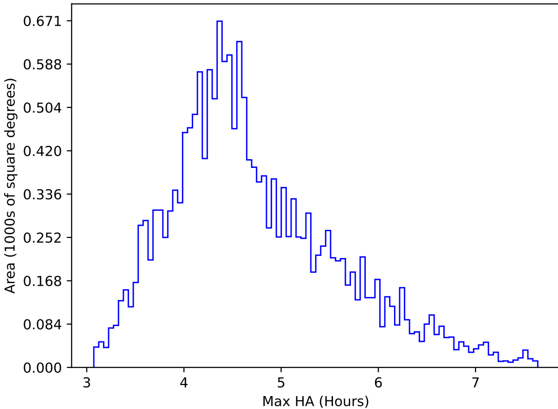
weather_cloudso10v3.4_10yrs WFD y band: Max HA
