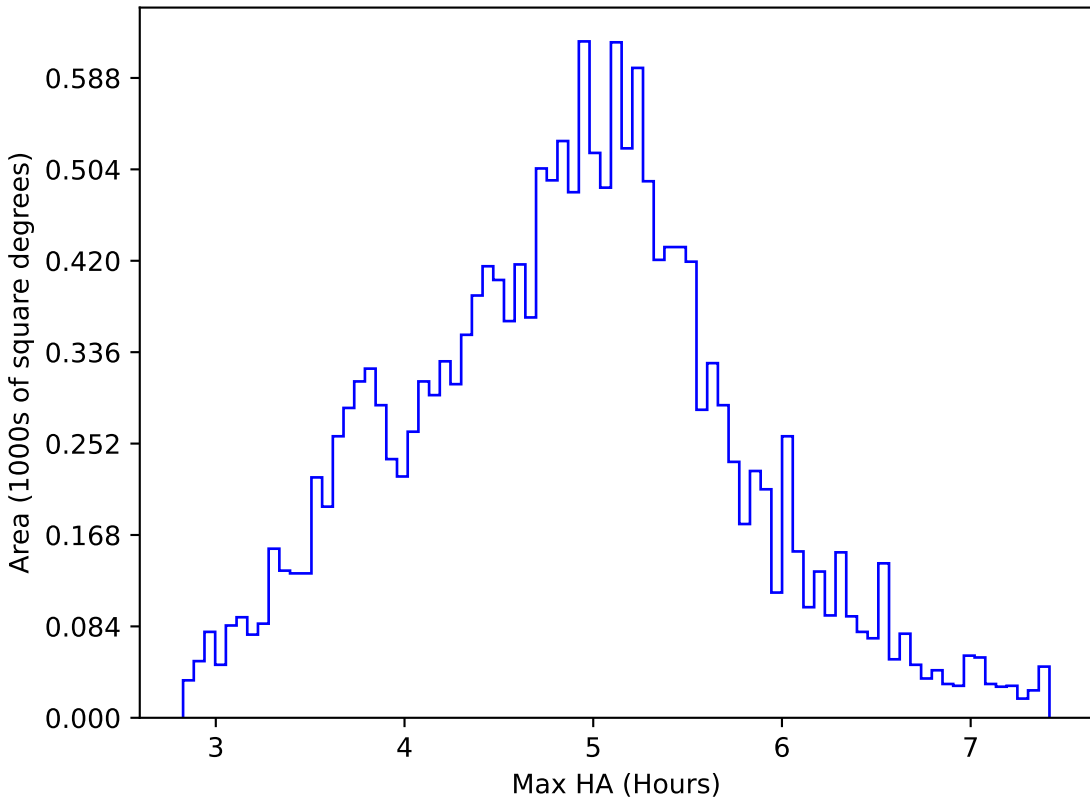
weather_cloudso10v3.4_10yrs WFD i band: Max HA
