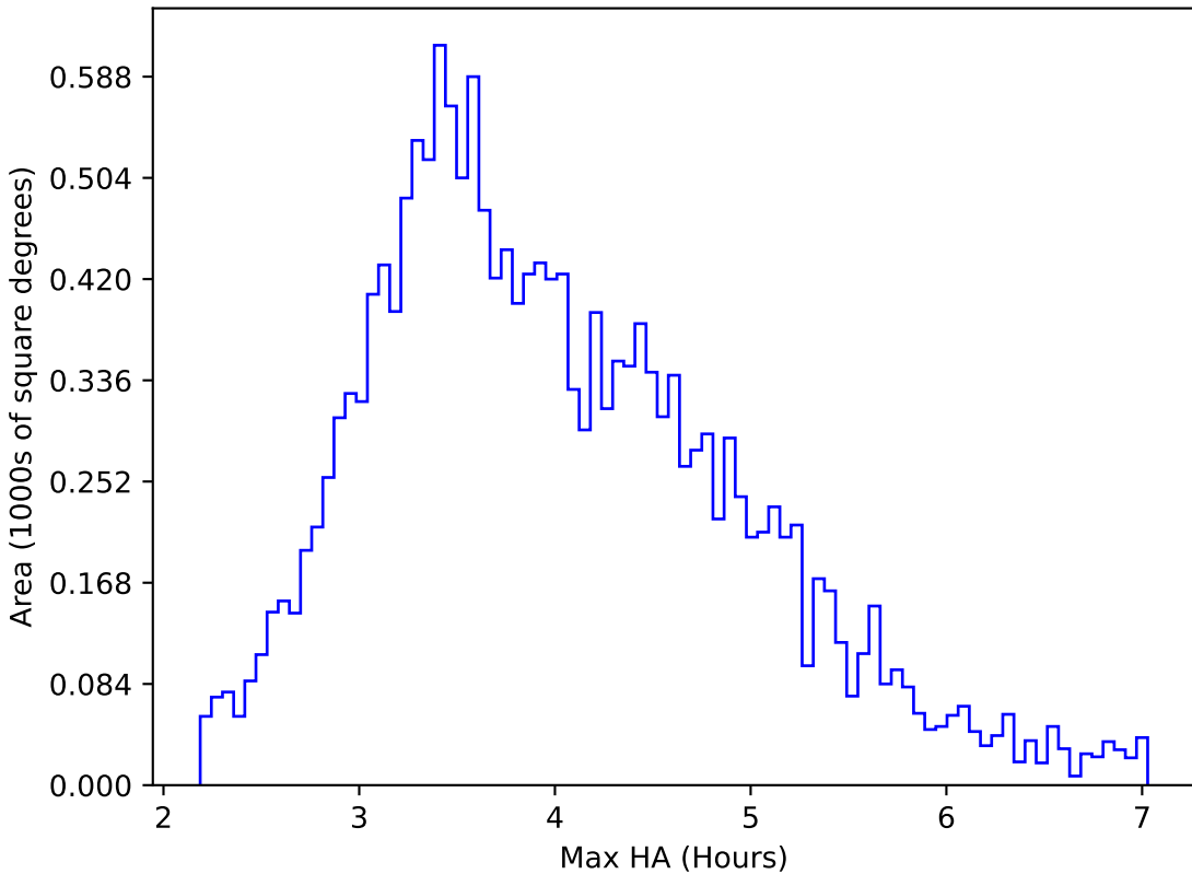
weather_cloudso10v3.4_10yrs WFD g band: Max HA
