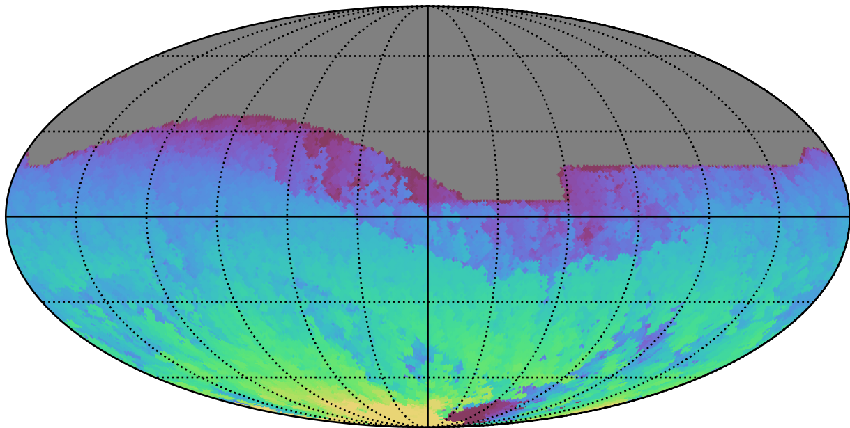
weather_cloudso10v3.4_10yrs All sky z band: Max HA
