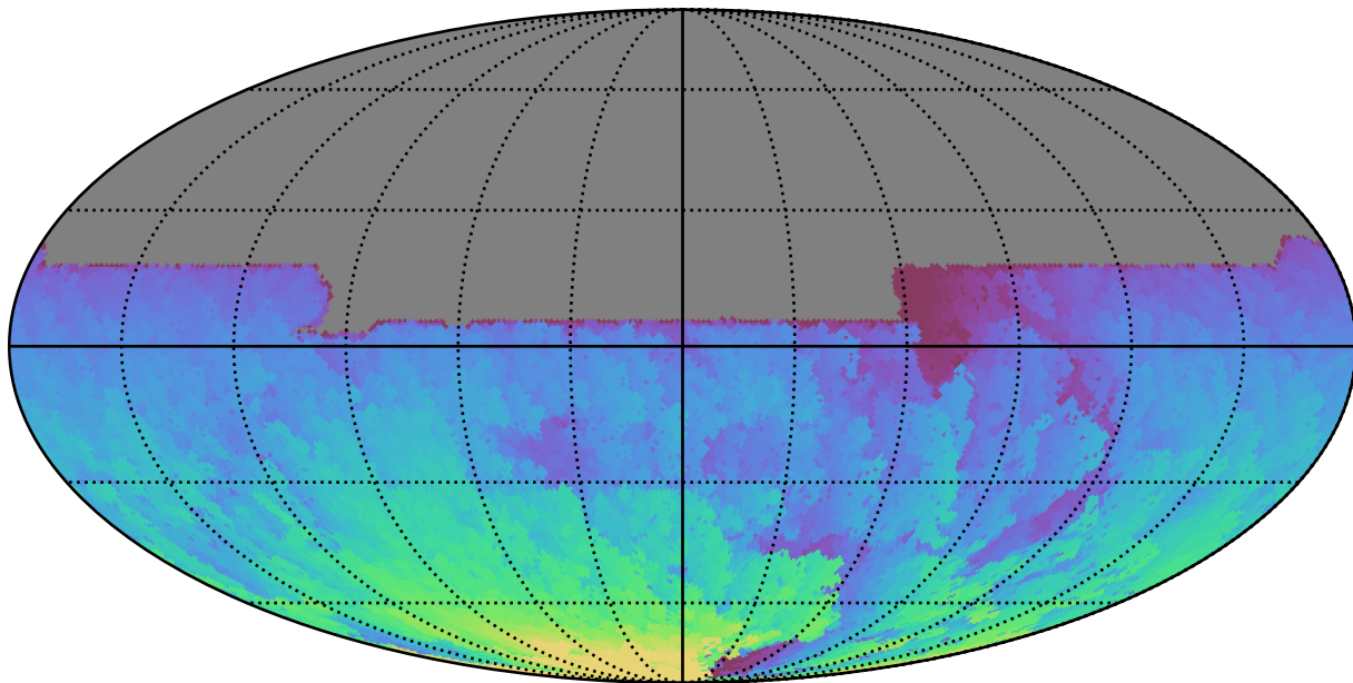
weather_cloudso10v3.4_10yrs All sky y band: Max HA
