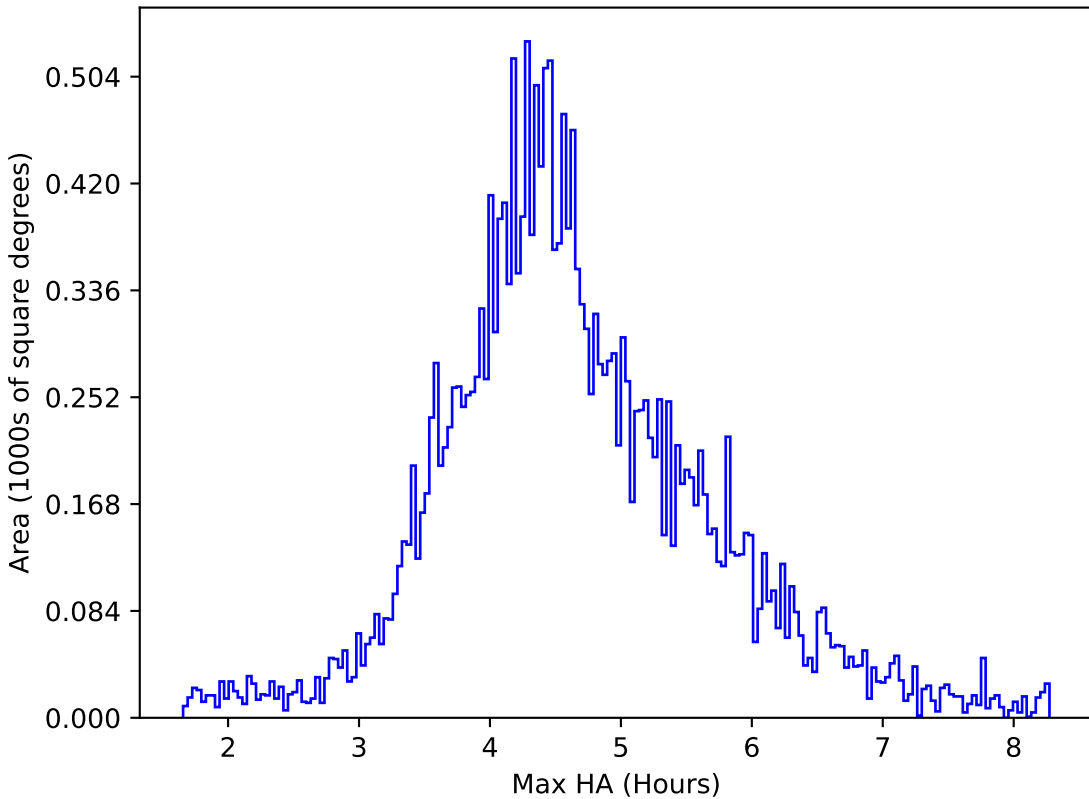
weather_cloudso10v3.4_10yrs All sky y band: Max HA
