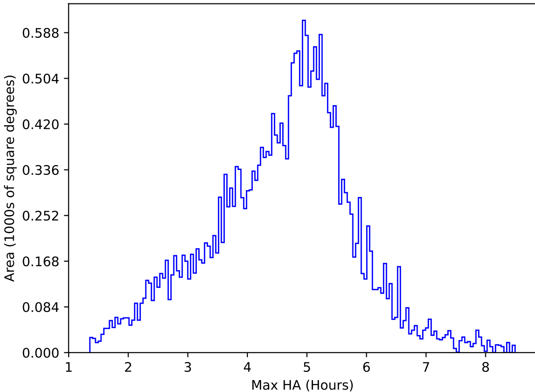
weather_cloudso10v3.4_10yrs All sky i band: Max HA
