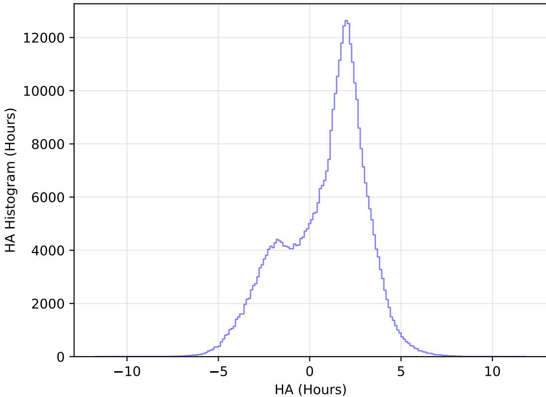
weather_cloudso10v3.4_10yrs WFD y band: HA Histogram
