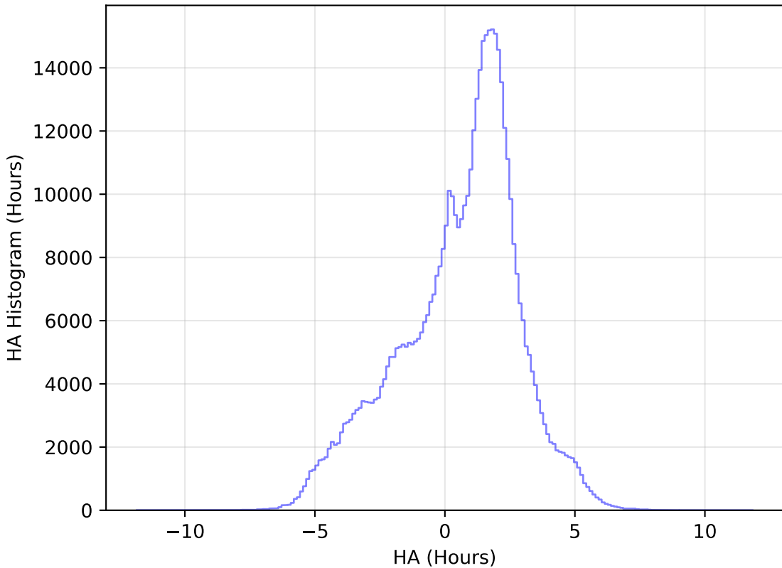
weather_cloudso10v3.4_10yrs WFD i band: HA Histogram
