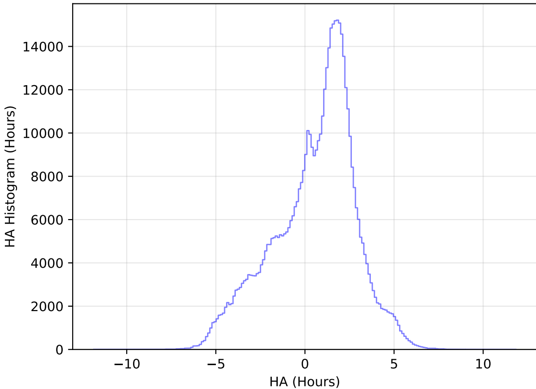
weather_cloudso10v3.4_10yrs All sky i band: HA Histogram
