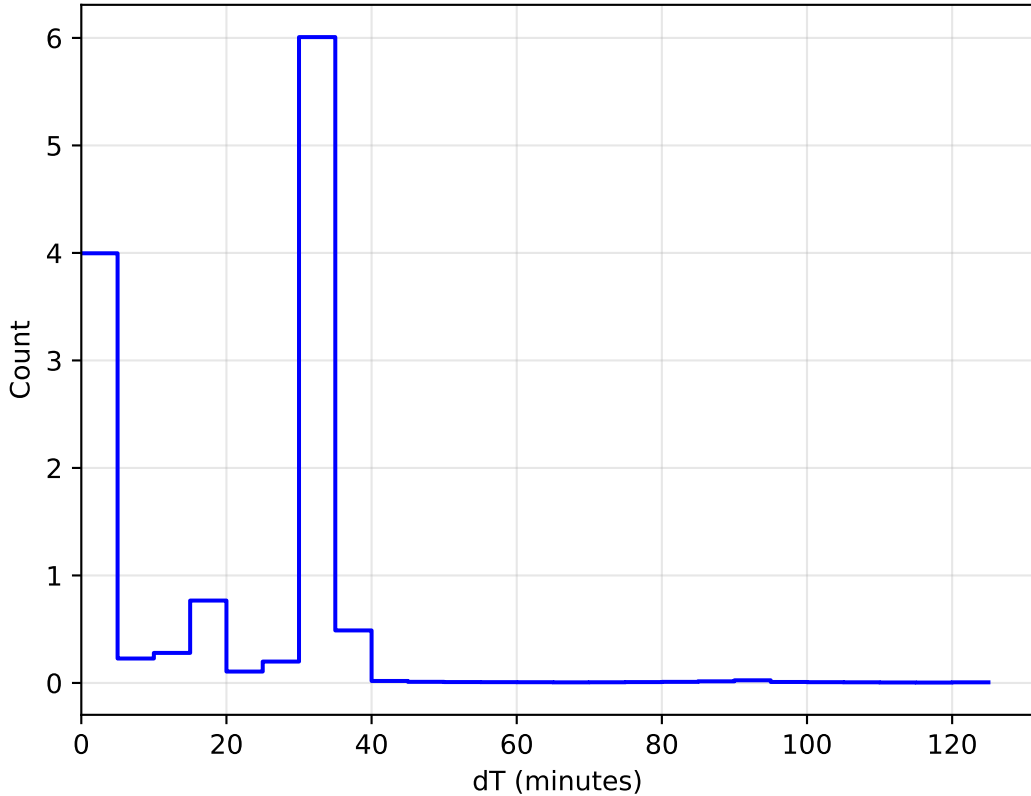
weather_cloudso10v3.4_10yrs WFD: DeltaT Histogram
